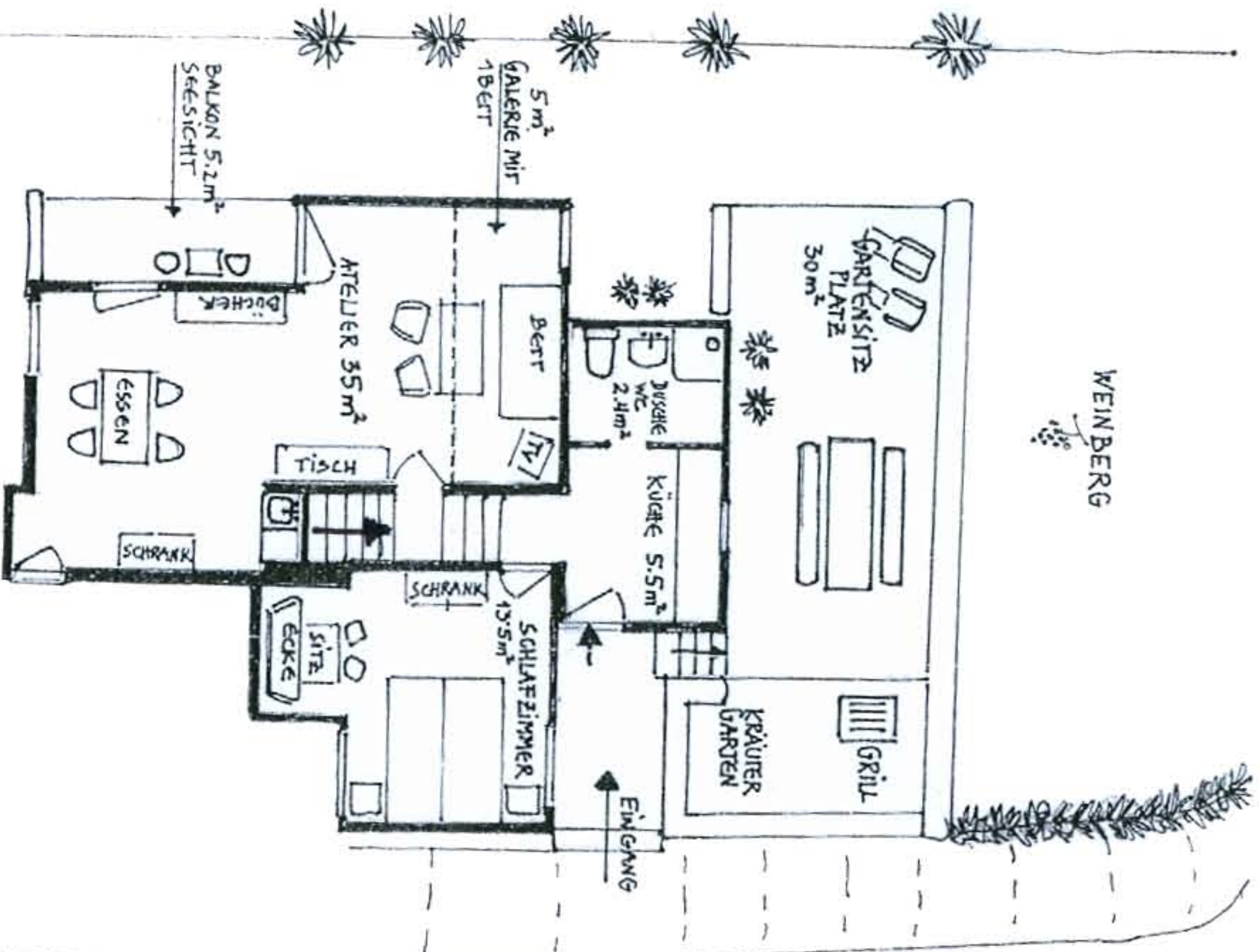
GRUNDRISS CASA DELL'ARTISTA WEINBERGSEITE TOTAL CA. 65 m² + GARTEN CA 50 m²
