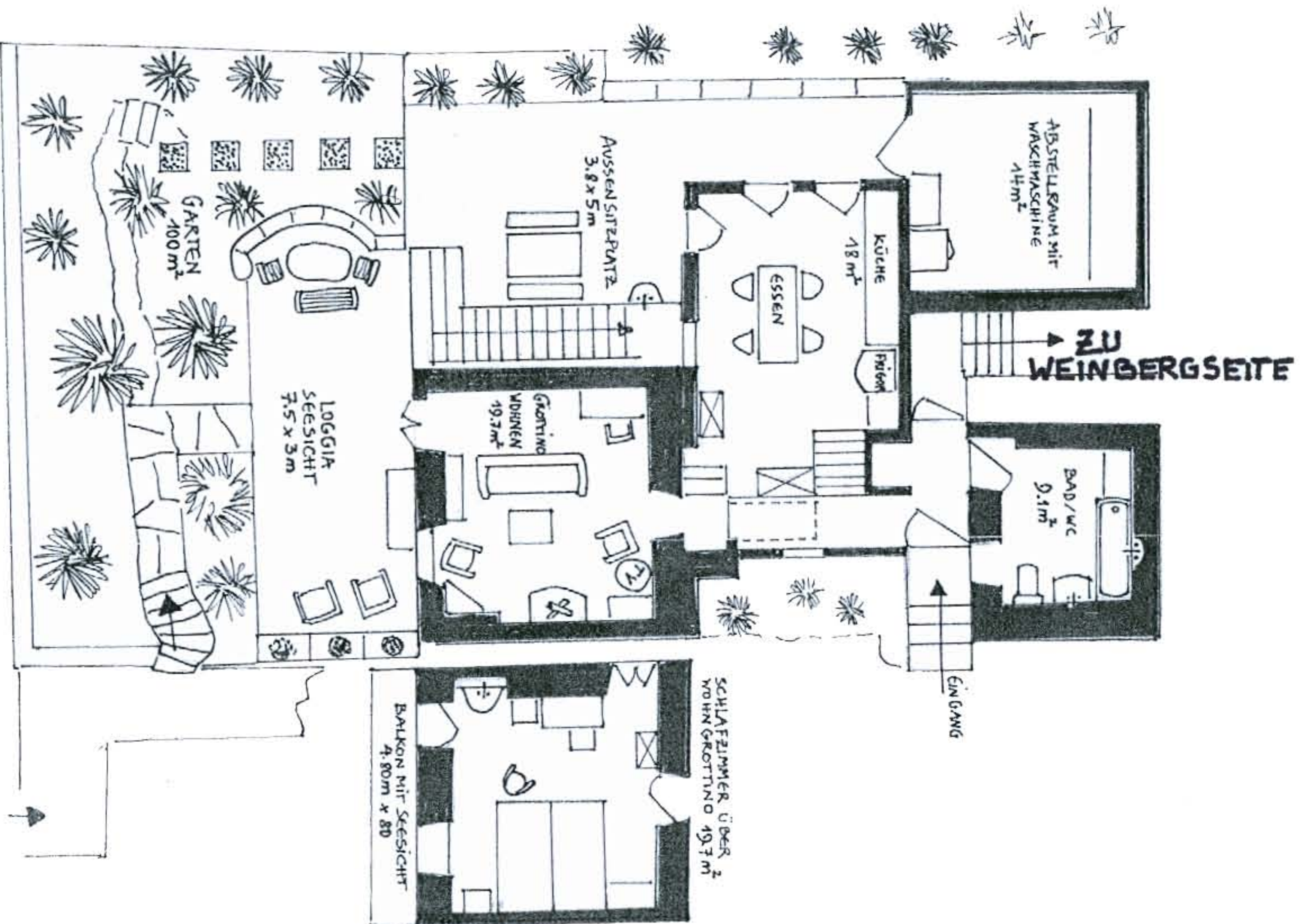
GRUNDRISS CASA DELL'ARTISTA SEESEITE TOTAL CA 76 m² + GARTEN CA. 100 m²
